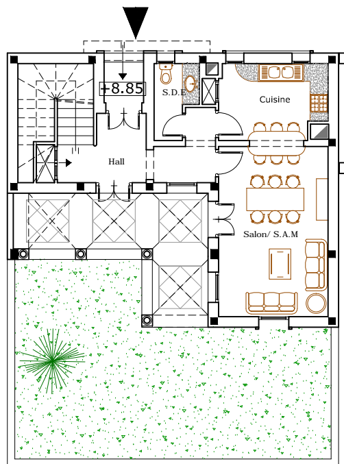
PLAN R.D.C
